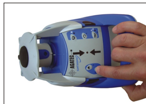
GAT220HV je vybavený elektronickou libelou na poloautomatické vytyčovanie zvislých rovín
